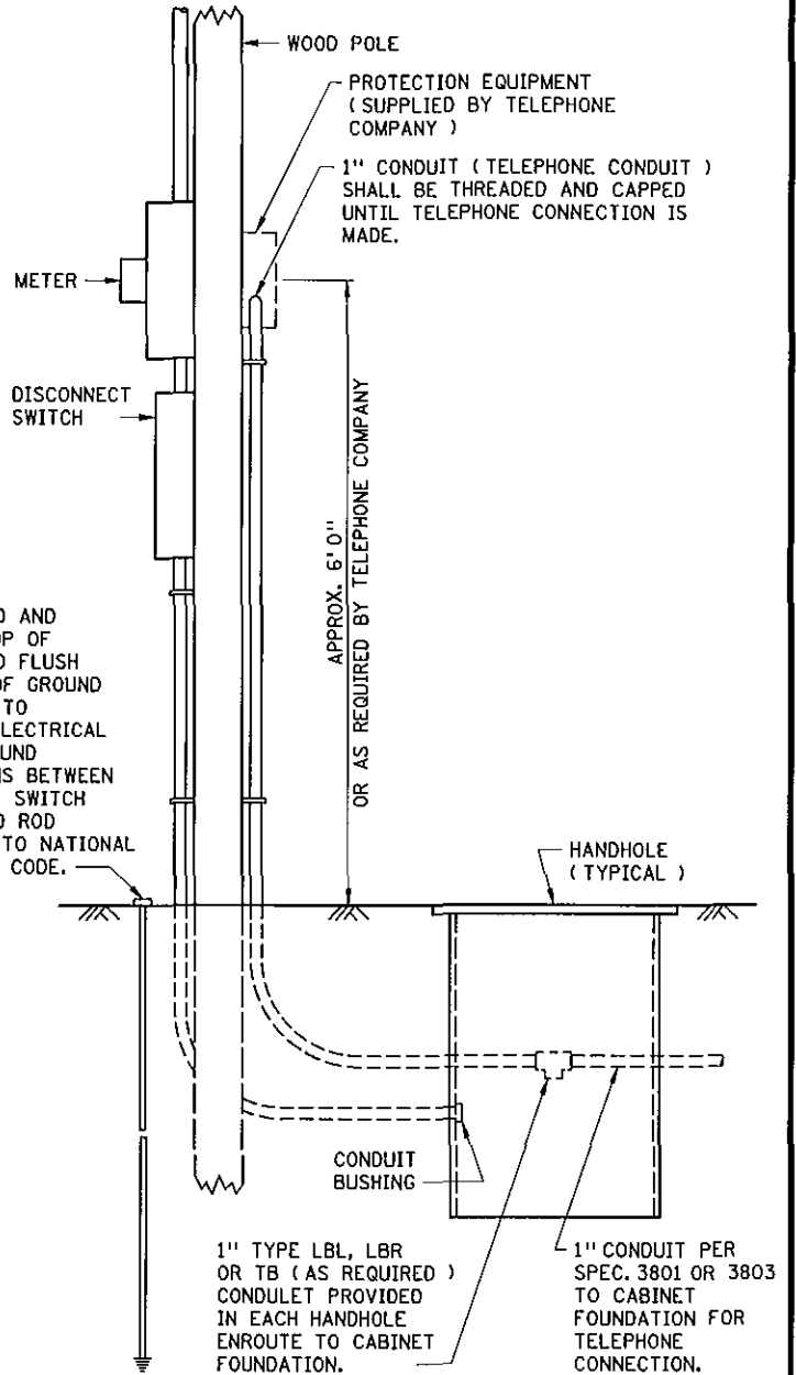
ELEVATION
