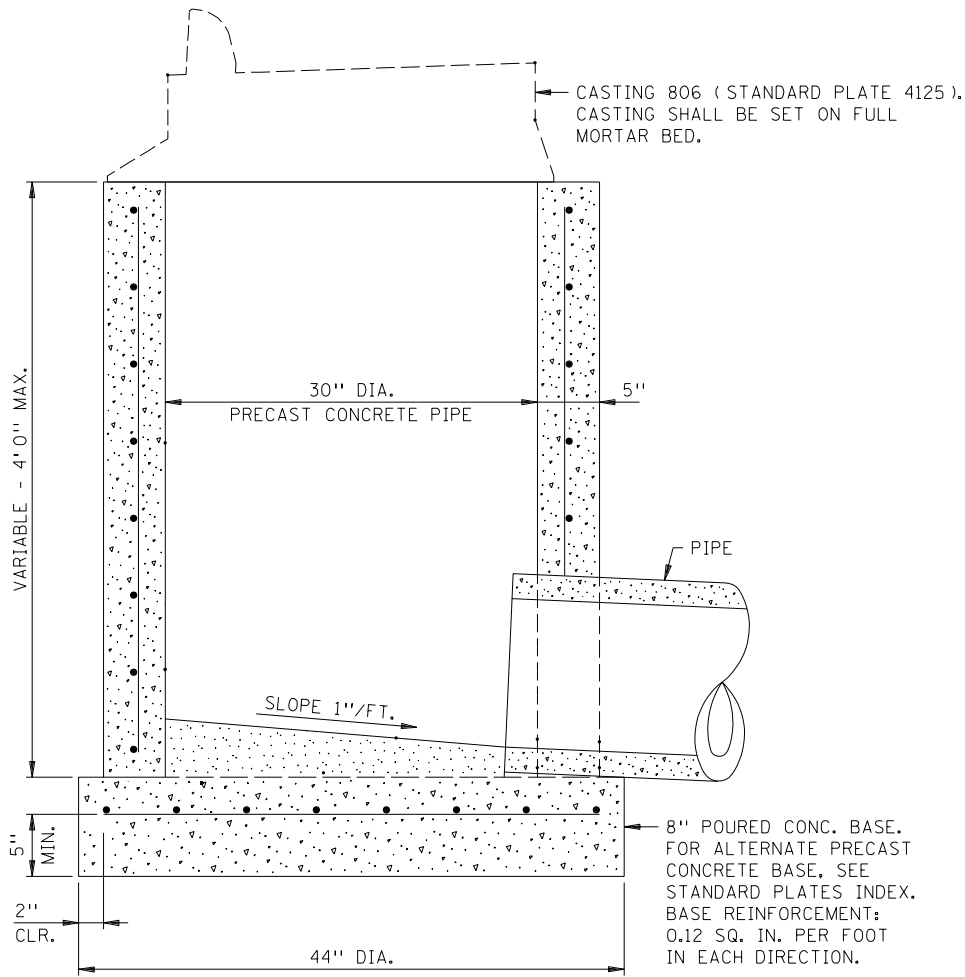
SECTION A-A
