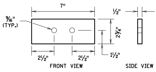
YOKE SPACER
