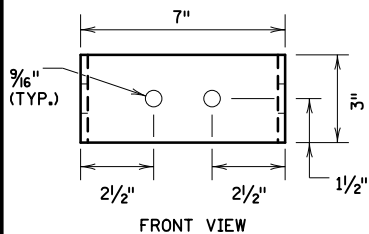
YOKE
